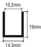
cat.nr. SDCD3812XX Lengte: 3,65m Glasdikte: 10mm
