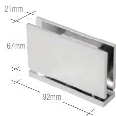
cat.nr. CAR01XX Montage aan bovenzijde of onderzijde Kan worden bevestigd aan de Deluxe bovenrailset
