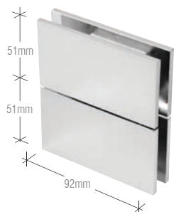
cat.nr. CAR02XX Glas-glas bevestiging
