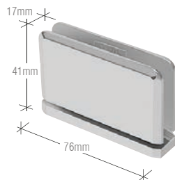
cat.nr. JRPPH01XX Montage aan bovenzijde of onderzijde
