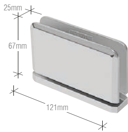
cat.nr. SRPPH01XX Montage aan bovenzijde of onderzijde
