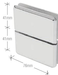
cat.nr. JRPPH02XX Glas-glas bevestiging
