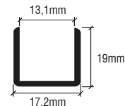
cat.nr. SDCD1212XX Lengte: 3,65m Glasdikte: 12mm
