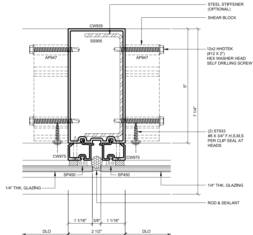
INT. VERT. PLAN
